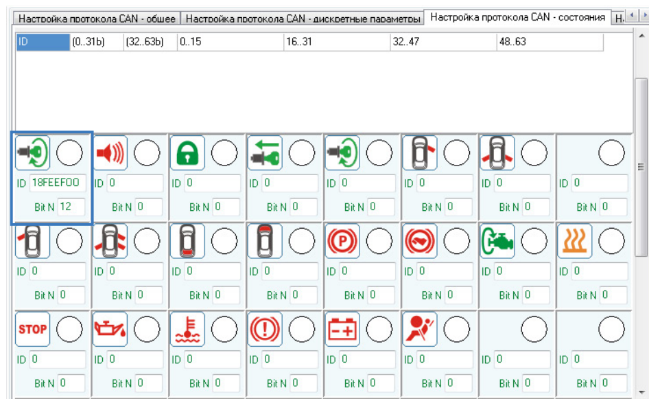
Рис.53. Вкладка «Настройка протокола CAN – состояния».
