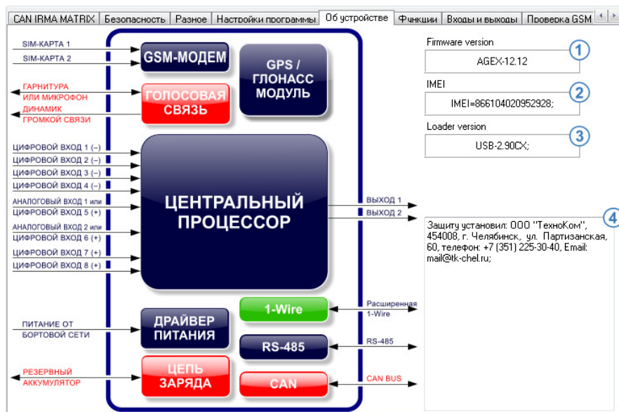
Рис.62. Вкладка «Об устройстве».
