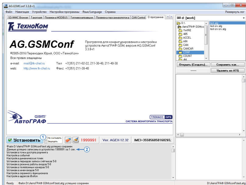
Рис.82. Запись настроек в прибор.
