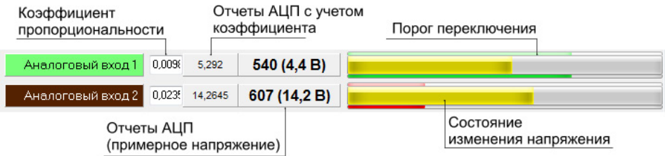
Рис.68. Состояние работы аналоговых входов.
