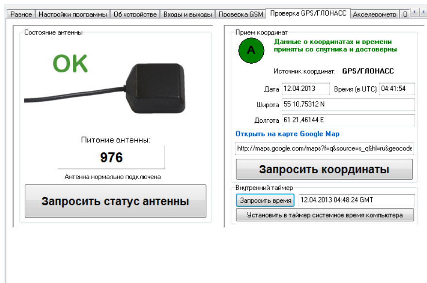
Рис.74. Вкладка Контроль. Проверка GPS/ ГЛОНАСС.
