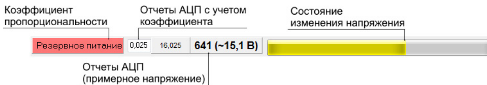
Рис.69. Резервное питание прибора.
