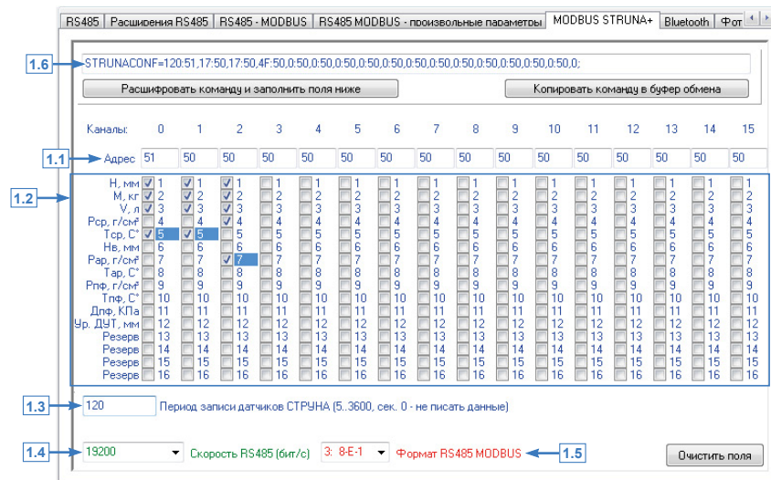
Рис.42. Вкладка «MODBUS STRUNA+».
