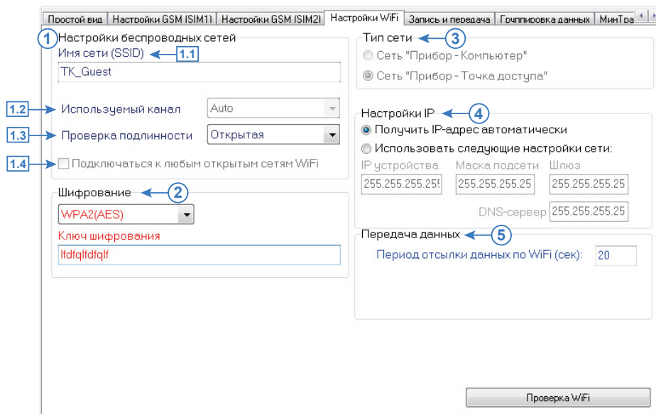
Рис.15. Настройки Wi-Fi.
