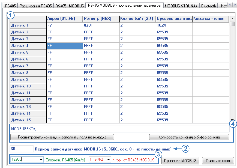
Рис.41. Вкладка «RS-485 произвольные параметры».
