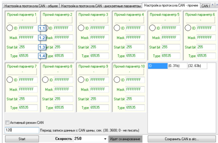
Рис.60. Вкладка «Настройка протокола CAN – прочее».
