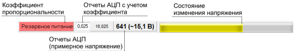
Рис.77. Резервное питание прибора.
