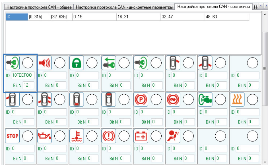
Рис.61. Вкладка «Настройка протокола CAN – состояния».
