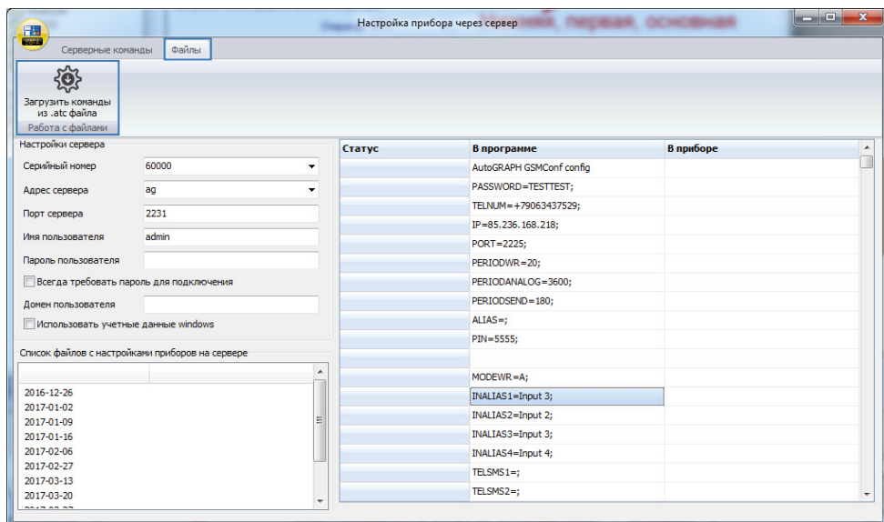
Рис.101. Загрузка списка команд из АТС файла.
