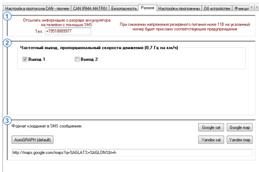
Рис.68. Вкладка «Разное».
