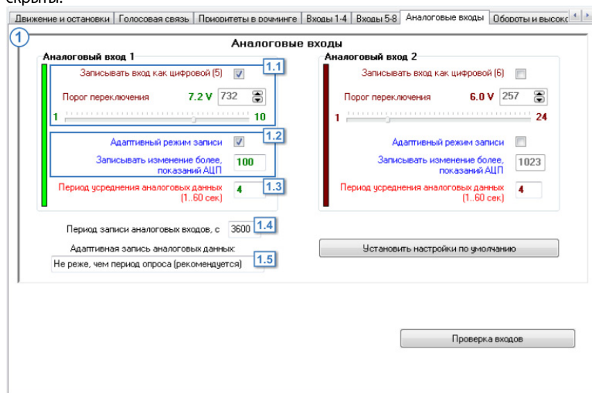
Рис.29. Аналоговые входы.
