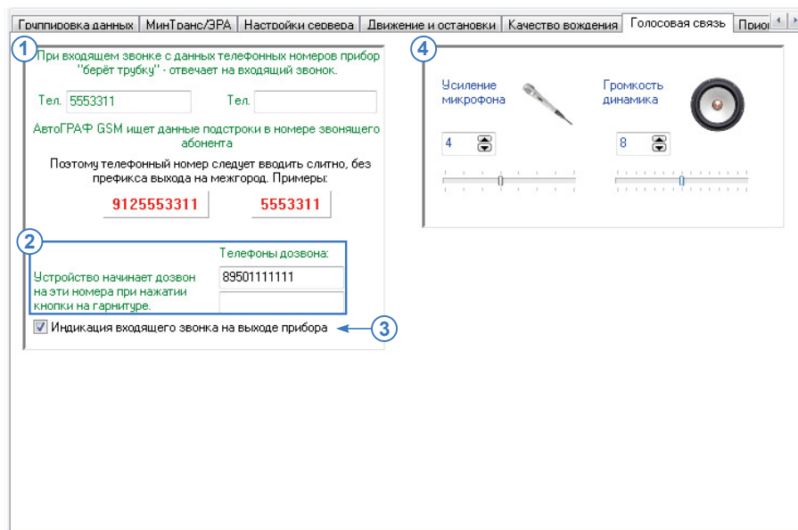
Рис.25. Голосовая связь.
