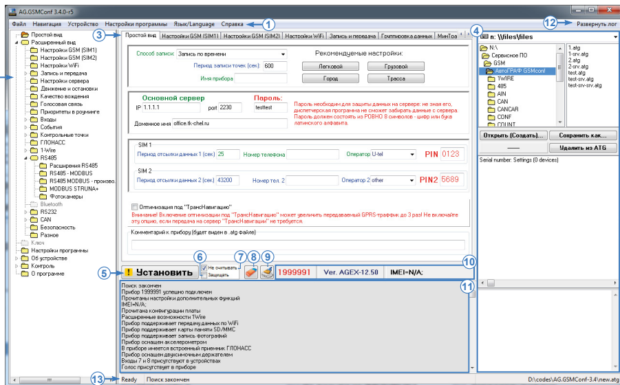
Рис.6. Интерфейс программы.
