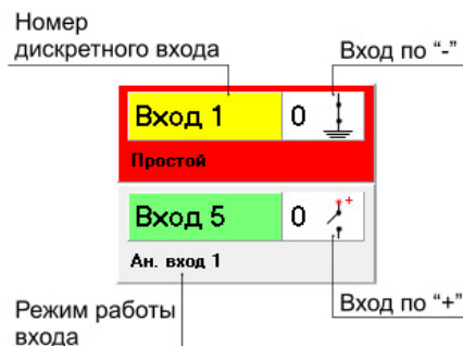
Рис.79. Цифровые входы.
