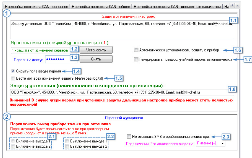
Рис.67. Вкладка «Безопасность».
