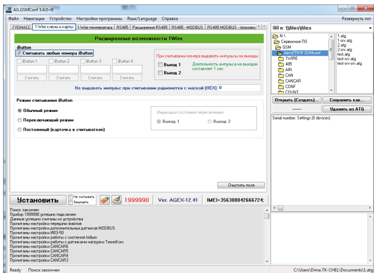
Рис.20. Настройка шины 1-Wire контроллера «АвтоГРАФ» на считывание любых номеров.
