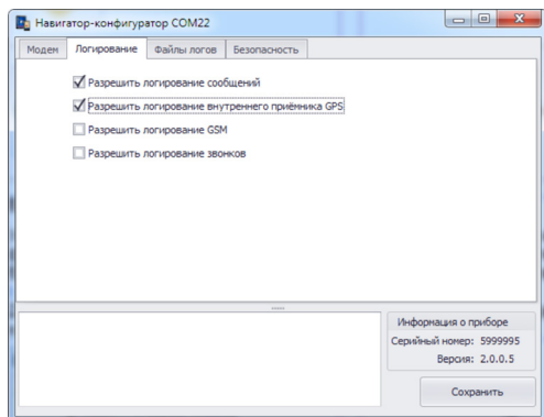
Рис.65. Вкладка «Логирование».
