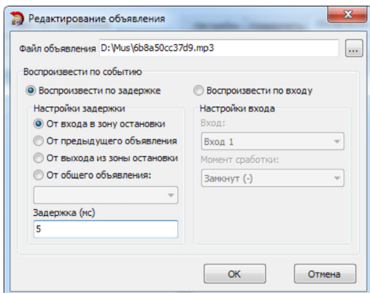
Рис.55. Редактирование объявления.
