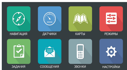
Рис.9. Главное меню.
