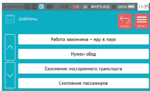
Рис.41. Шаблоны сообщений.
