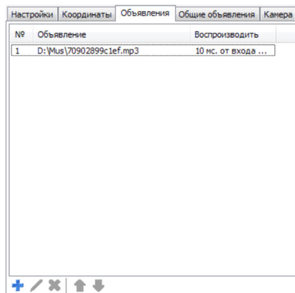
Рис.54. Объявления.
