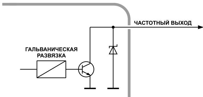
Рис.13. Внутренняя схема частотного выхода датчика «TKLS-L» варианта исполнения F-RS485.
