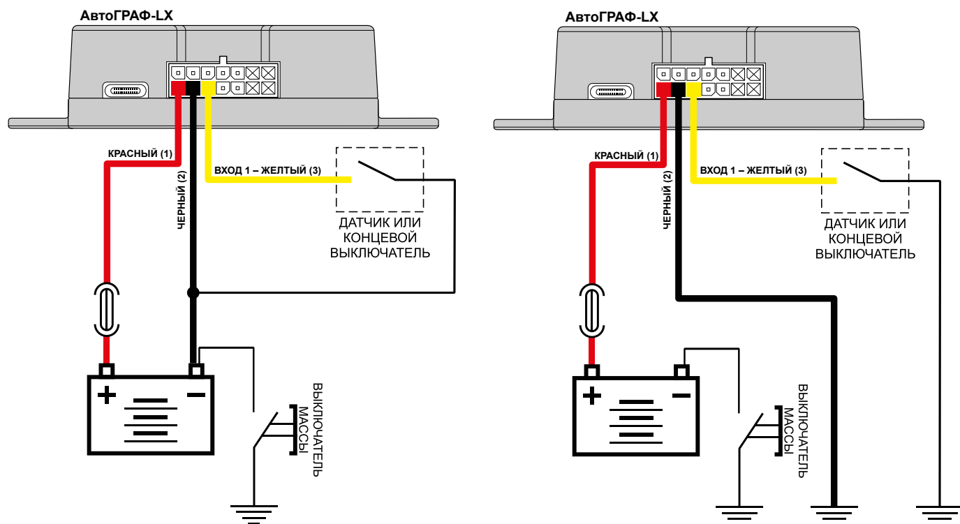
1 – с подтяжкой, подключение питания до выключателя массы
