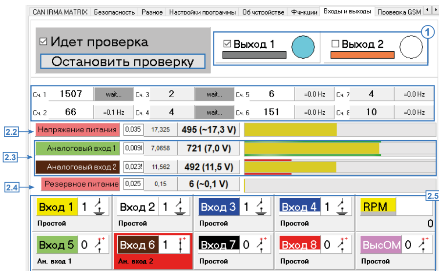
Рис.81. Вкладка «Контроль. Входы и выходы».
