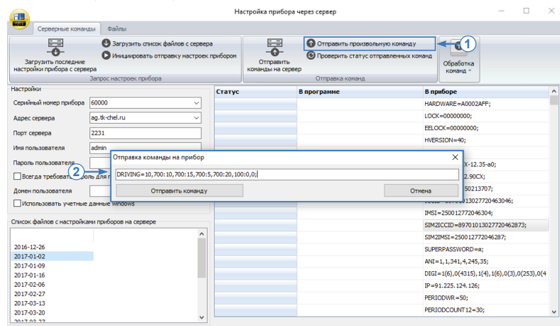
Рис.106. Отправка произвольной команды.
