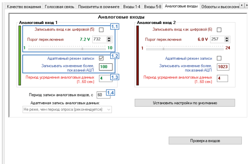
Рис.35. Аналоговые входы.
