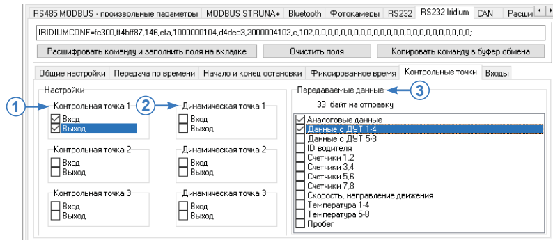
Рис.61. Вкладка «Контрольные точки» (RS232 Iridium).
