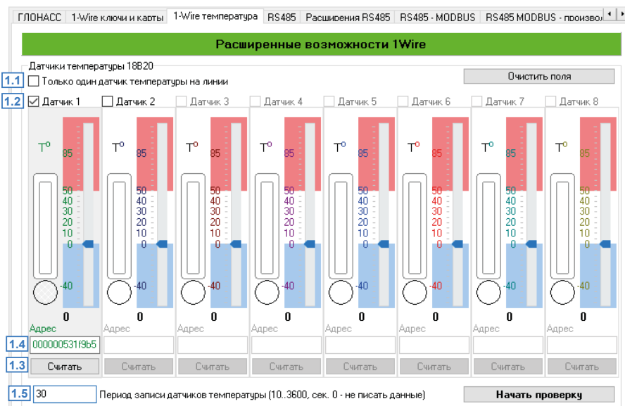
Рис.43. Вкладка «1-Wire температура».
