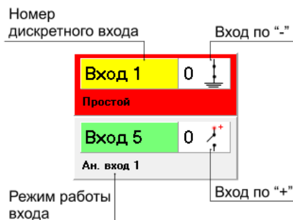
Рис.87. Цифровые входы.
