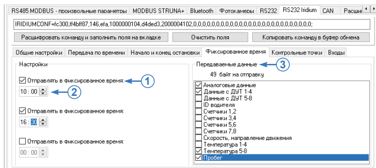
Рис.60. Вкладка «Фиксированное время» (RS232 Iridium).
