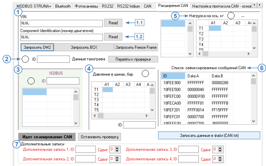
Рис.66. Вкладка «Расширения CAN».
