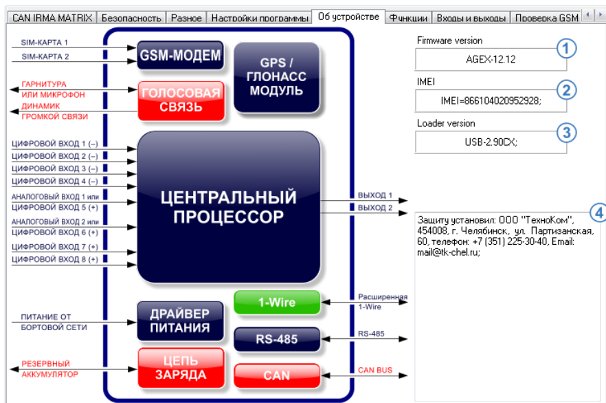
Рис.79. Вкладка «Об устройстве».
