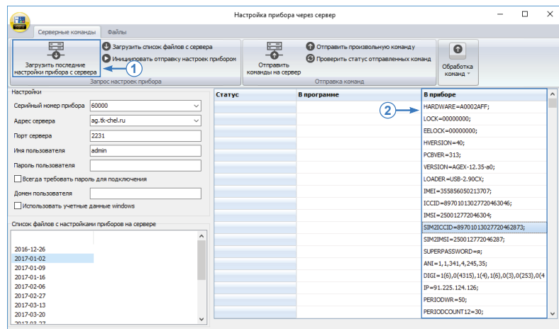
Рис.105. Загрузка последних настроек прибора с сервера.
