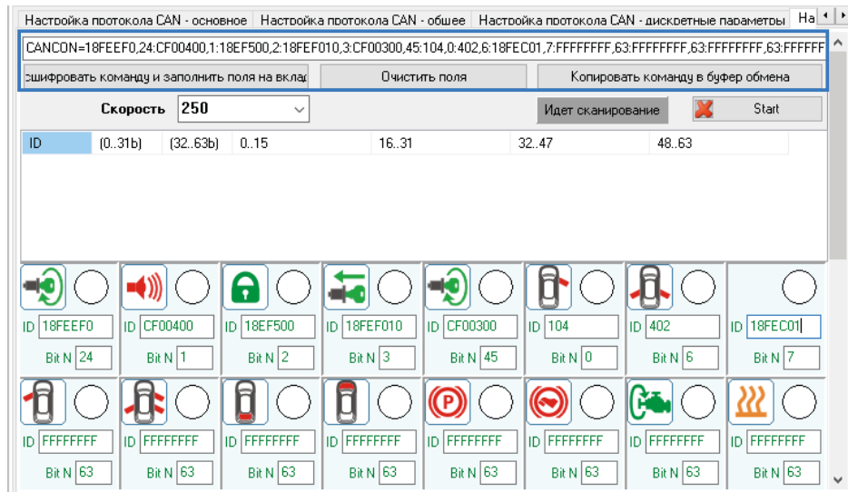
Рис.74. Команда удаленной настройки параметров состояния ТС с шины CAN.
