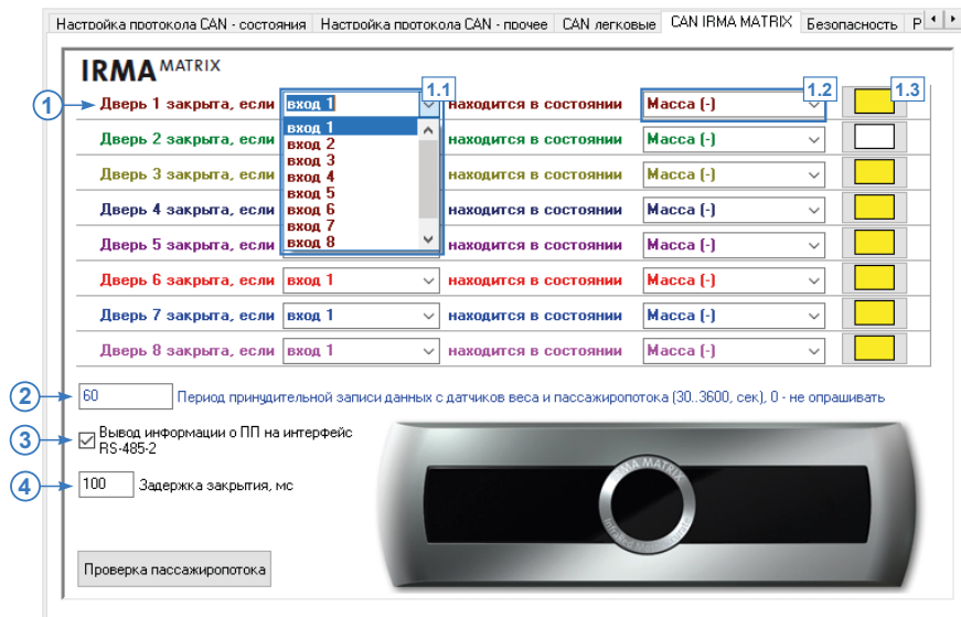
Рис.76. Вкладка «CAN IRMA MATRIX».
