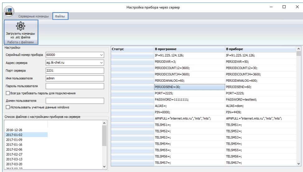
Рис.109. Загрузка списка команд из АТС файла.
