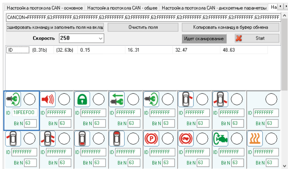
Рис.72. Вкладка «Настройка протокола CAN – состояния».
