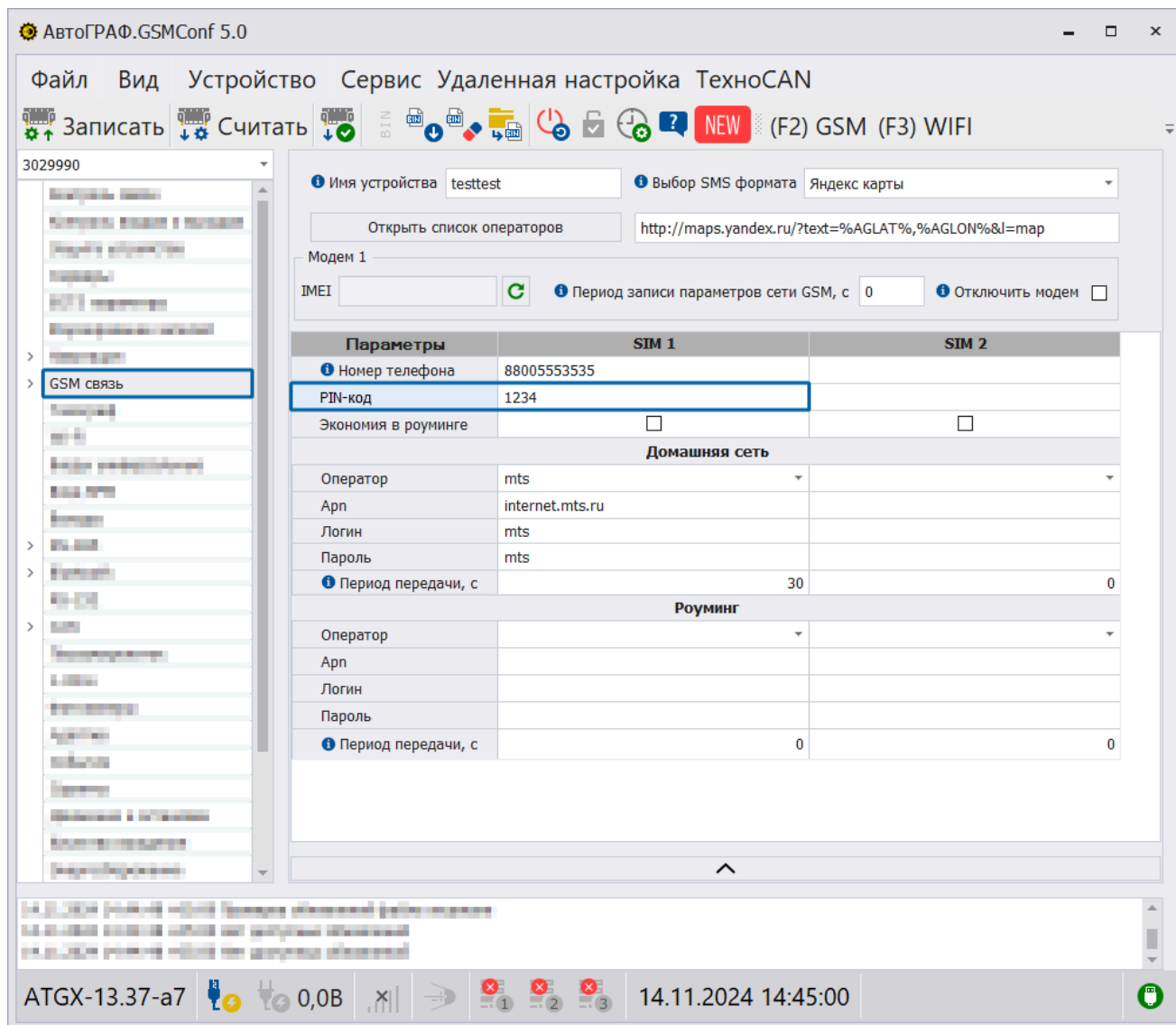
Рис.7. PIN-код
