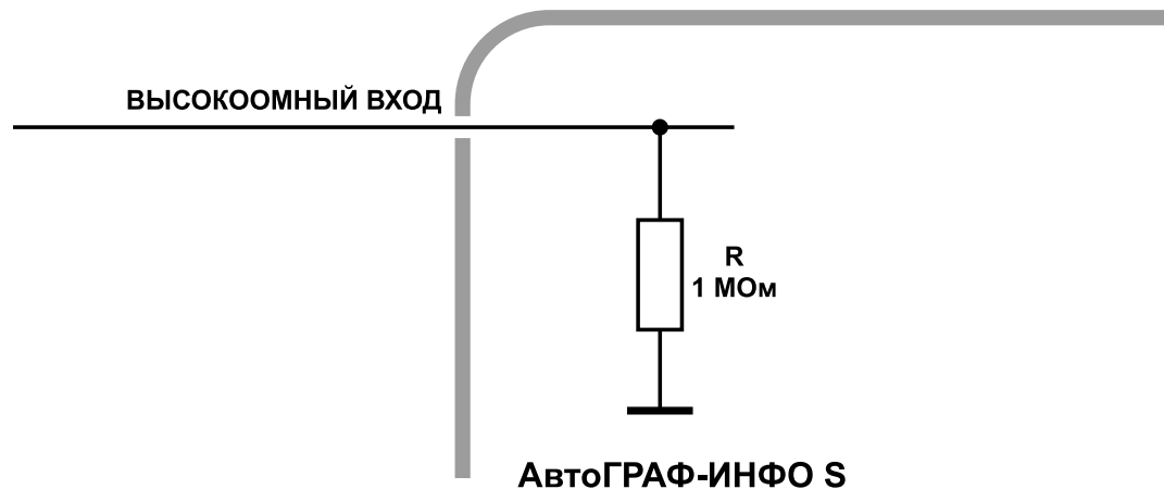
Рис.95. Внутренняя схема высокоомного входа
