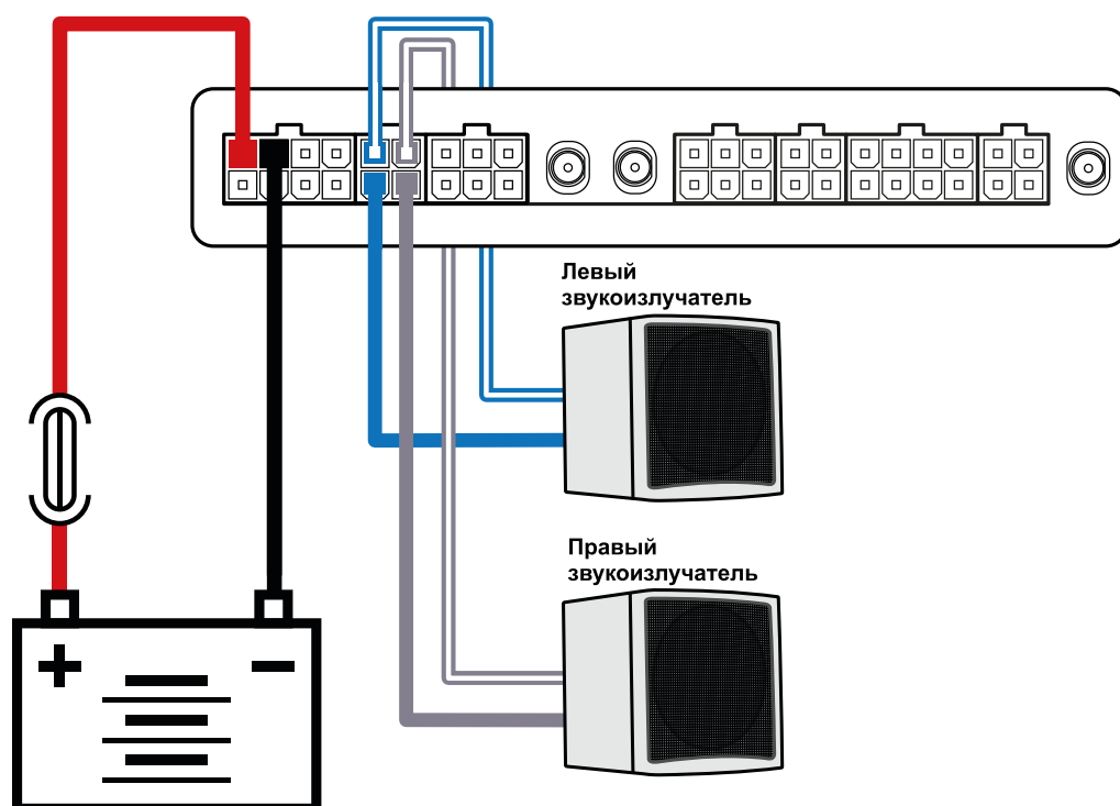
Рис.100. Подключение излучателя громкой связи
