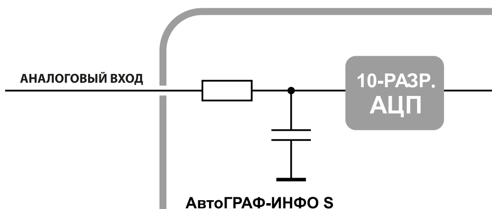
Рис.98. Внутренняя схема аналоговых входов
