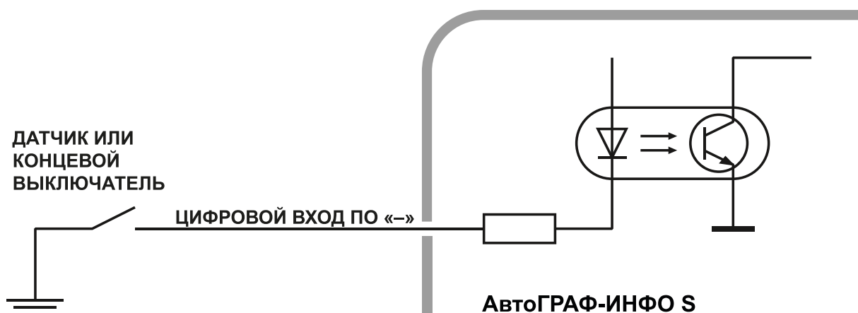
Рис.96. Внутренняя схема цифрового входа по «–»
