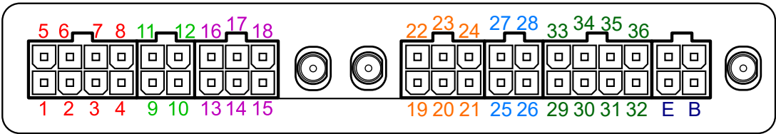
Рис.2. Интерфейсные разъемы контроллера АвтоГРАФ-ИНФО S
