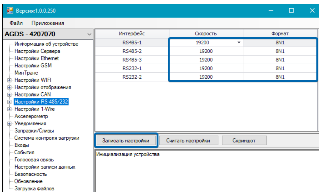
Рис.83. Настройка интерфейса шины RS-485/232
