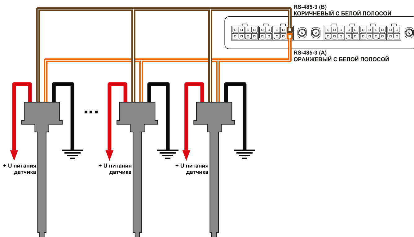
Рис.105. Структурная схема подключения датчиков уровня топлива
