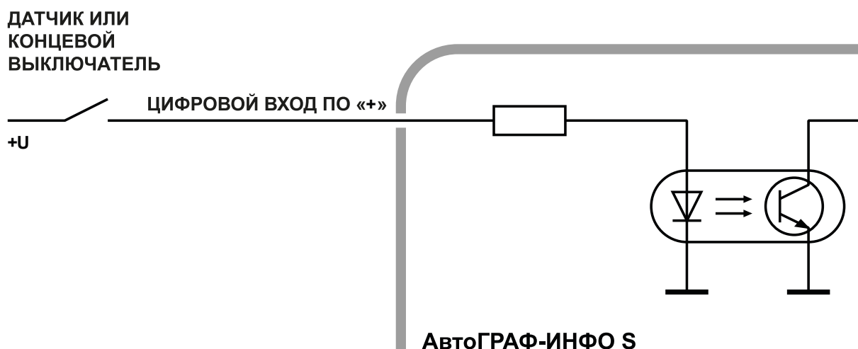
Рис.97. Внутренняя схема цифрового входа по «+»
