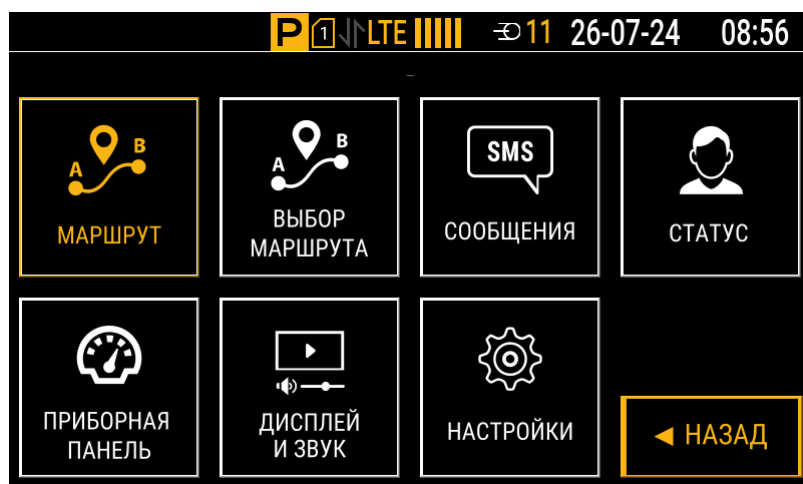
Рис.9. Главное меню
