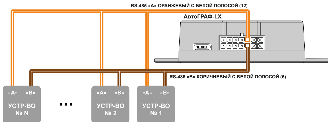
Рис.12. Схема подключения по шине RS-485
