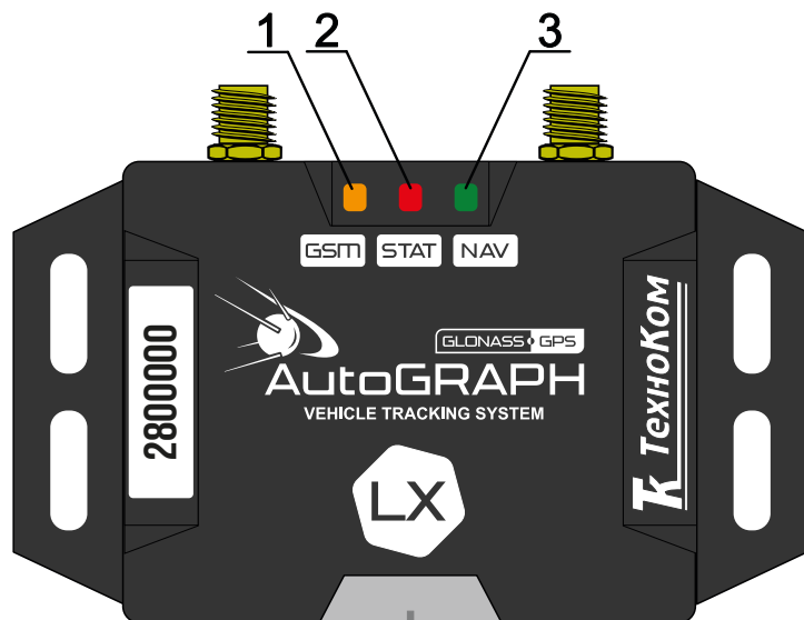
Рис.5. Индикация контроллера
