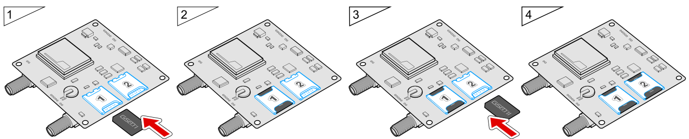
Рис.2. Установка SIM-карты
