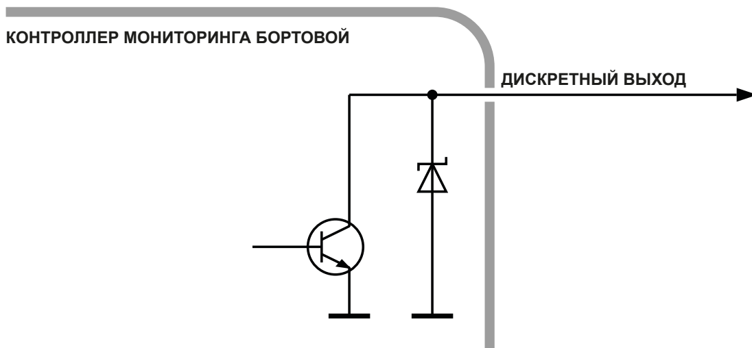
Рис.10. Внутренняя схема выхода
