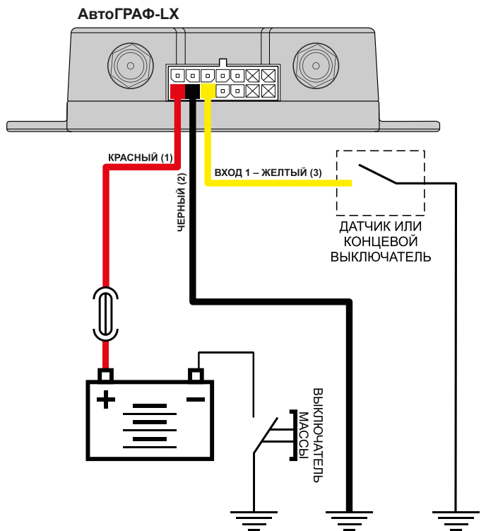
2 — с подтяжкой, подключение питания после выключателя массы
