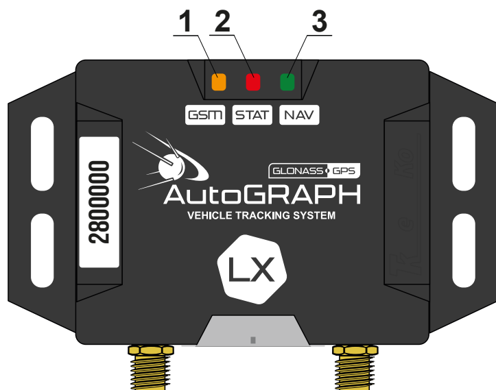
Рис.5. Индикация контроллера
