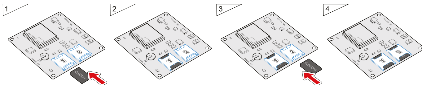
Рис.2. Установка SIM-карты
