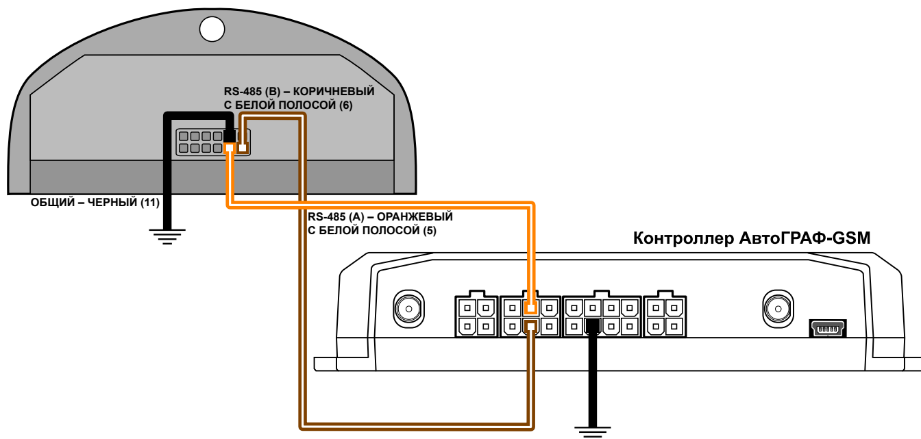
Рис.7. Схема подключения устройств по шине RS-485
