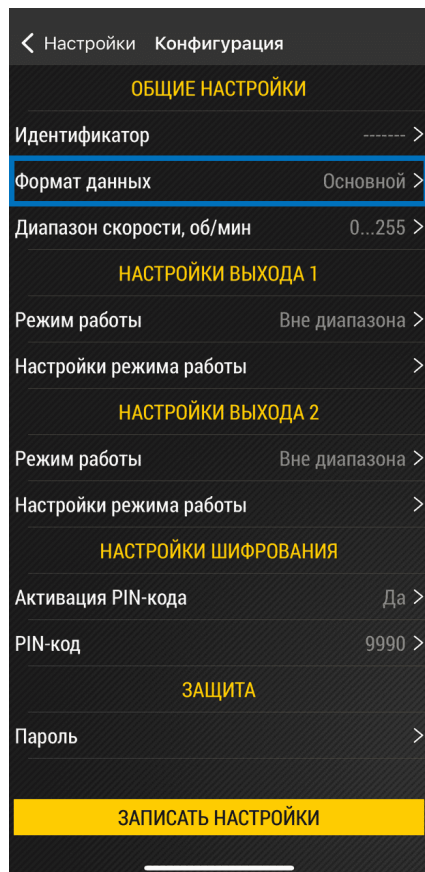
Рис.17. Формат данных
