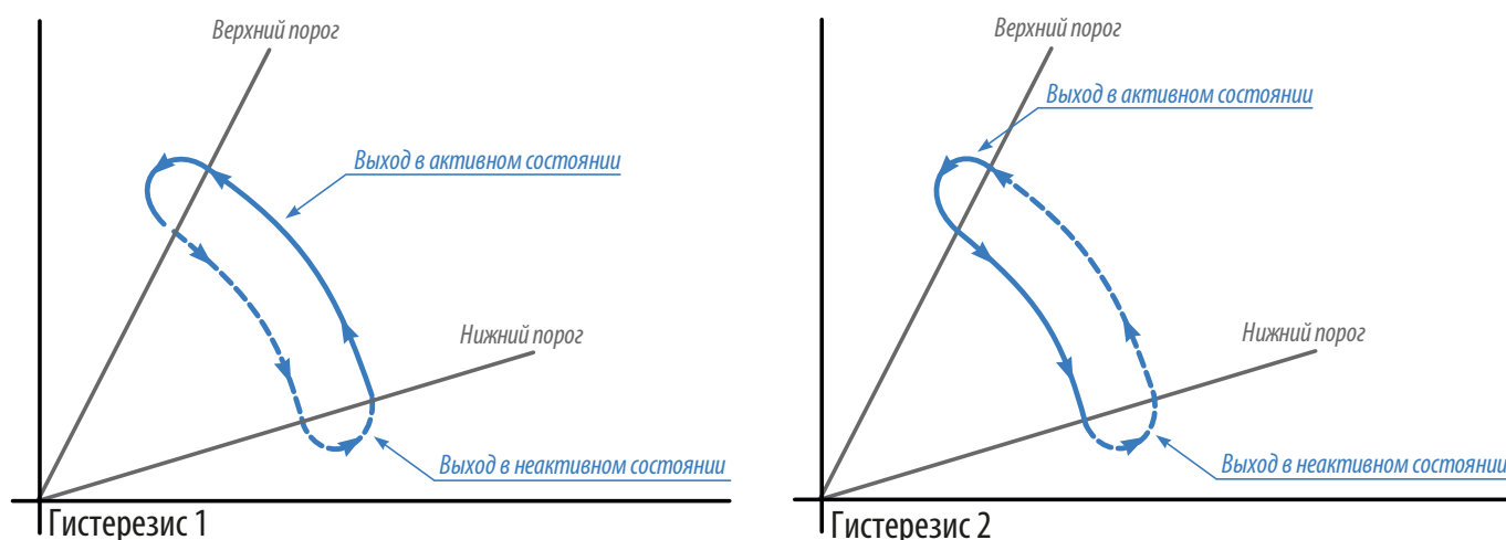
Рис.24. Порядок переключения выходов в режимах «Гистерезис 1» и «Гистерезис 2»
