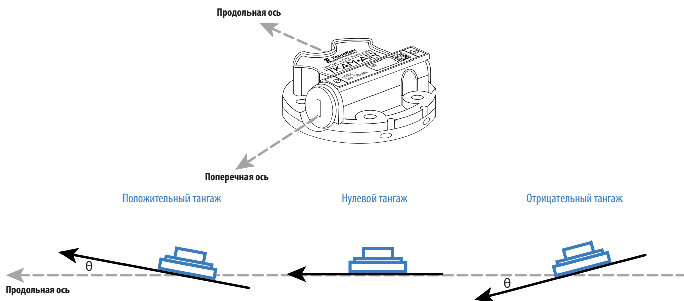
Рис.30. Измерение угла наклона относительно продольной оси датчика
