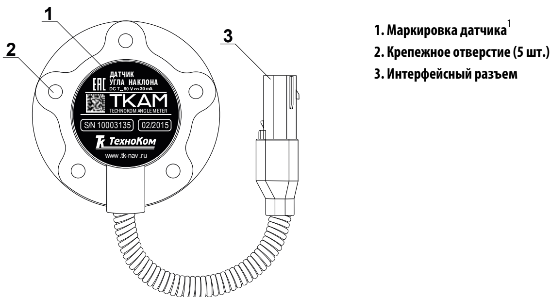
Рис.2. Составные части датчика
