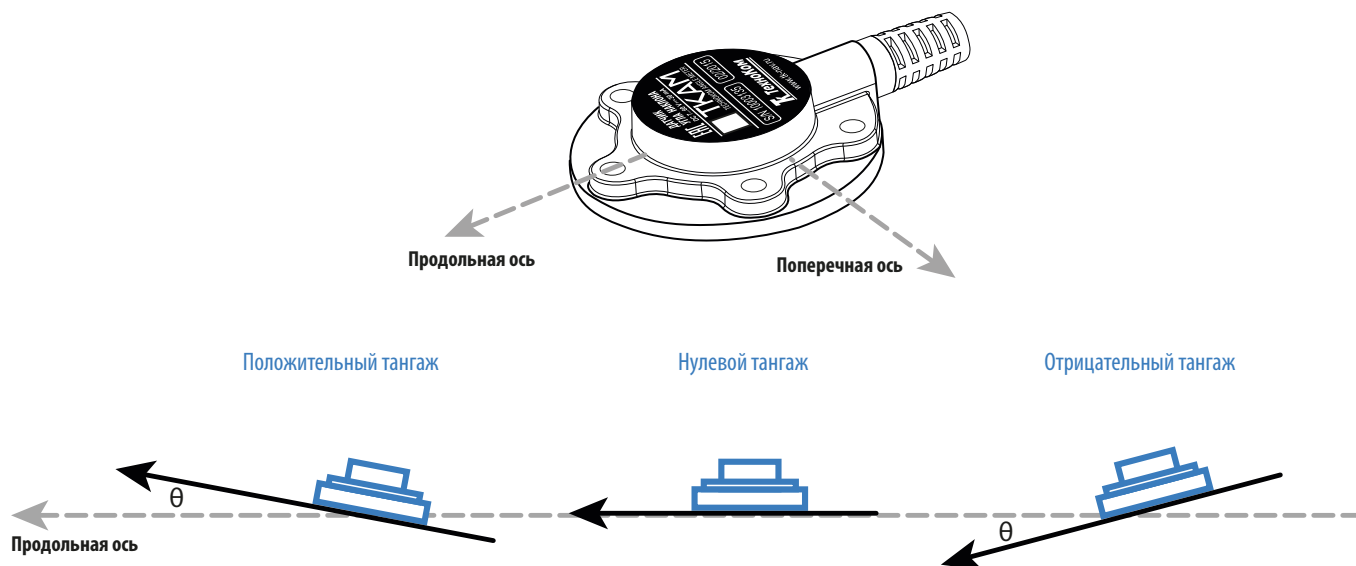
Рис.12. Измерение угла наклона относительно продольной оси датчика
