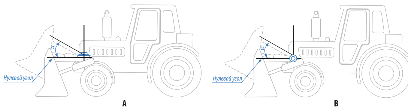
Рис.4. Пример установки датчика угла
