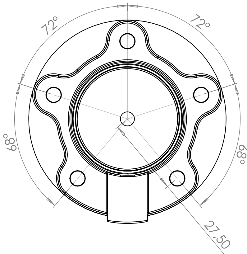
Рис.36. Расположение крепежных отверстий ТКАМ
