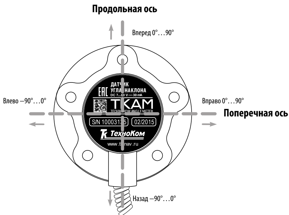
Рис.10. Оси датчика
