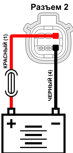
Рис.14. Схема подключения питания
