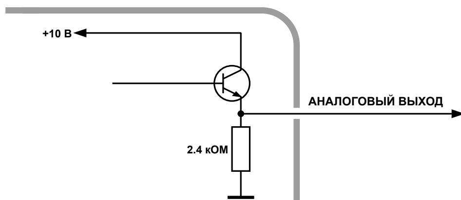
Рис.16. Внутренняя схема аналогового выхода
