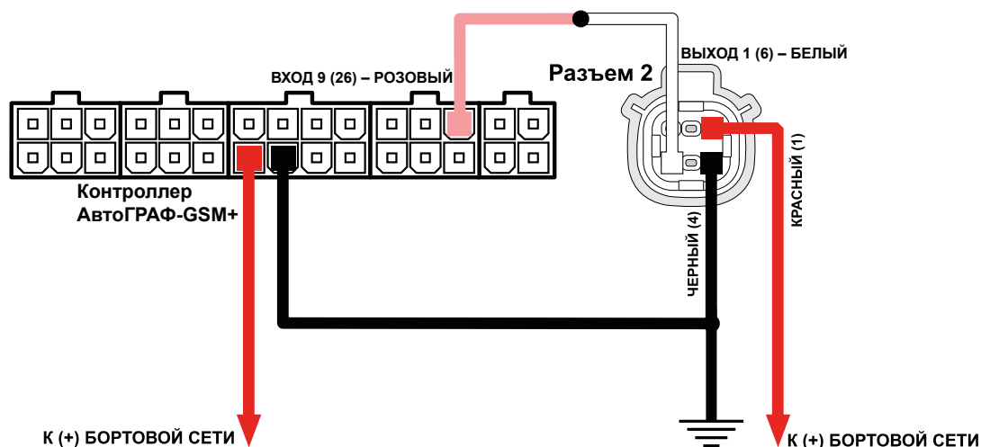
Рис.17. Структурная схема подключения аналогового выхода в цифровом режиме
