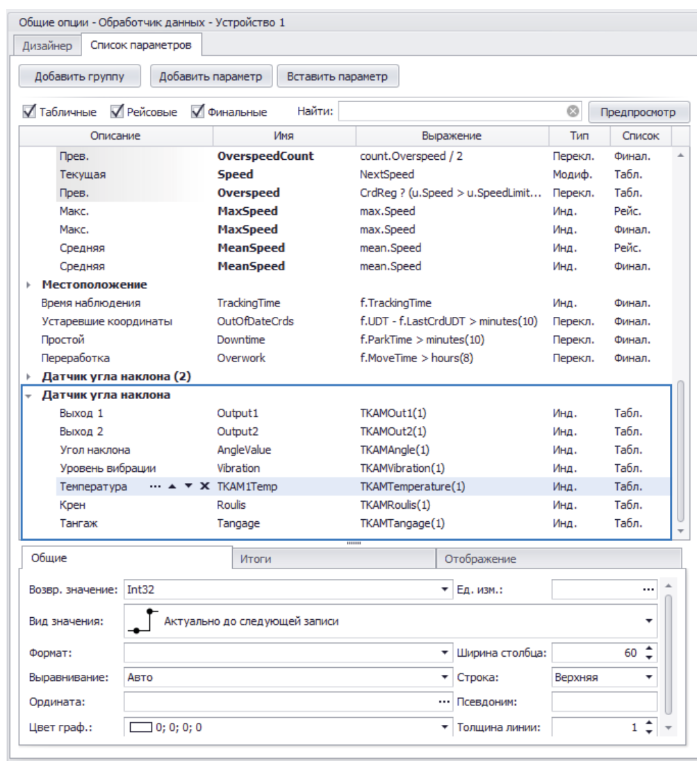
Рис.24. Показания датчика угла наклона ТКAM по каналу 1 в протоколе AGHIP
