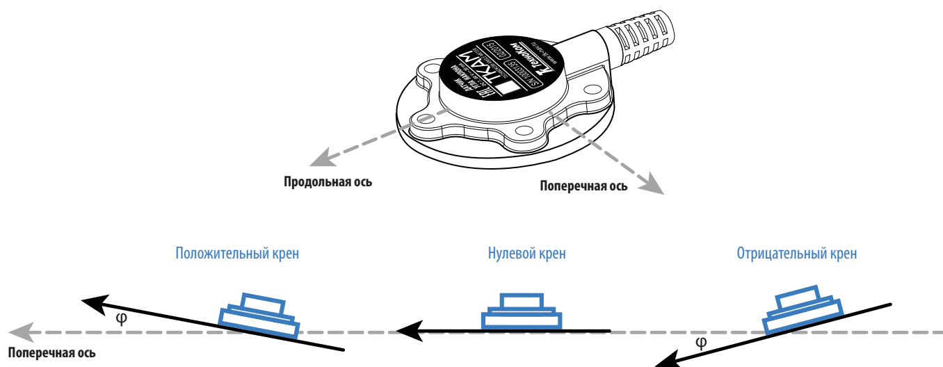
Рис.11. Измерение угла наклона относительно поперечной оси датчика
