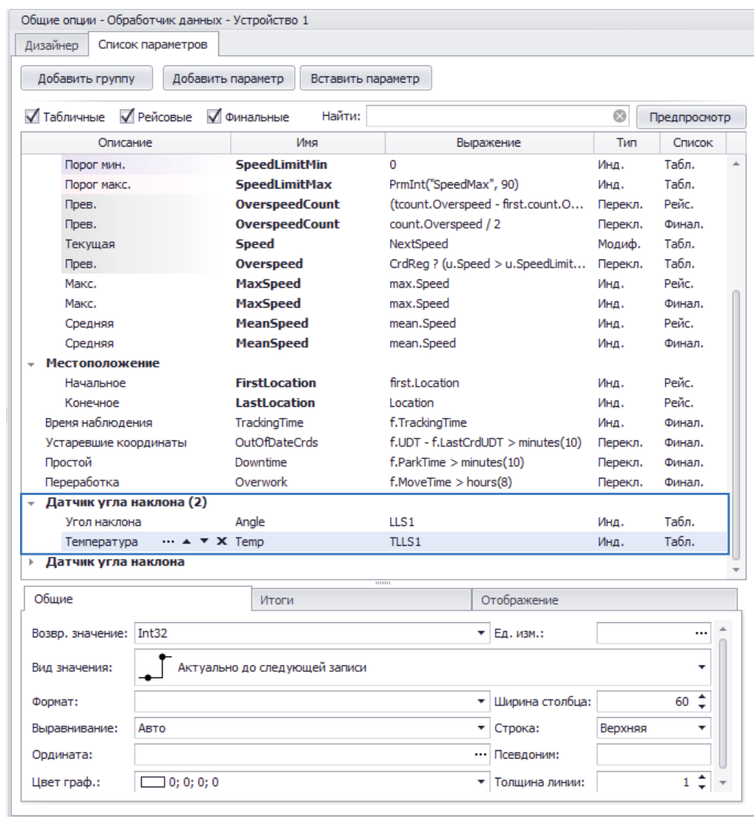
Рис.29. Показания датчика угла наклона ТКМ по каналу 1 в протоколе LLS
