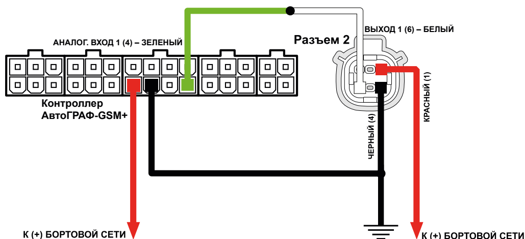
Рис.18. Структурная схема подключения аналогового выхода в аналоговом режиме
