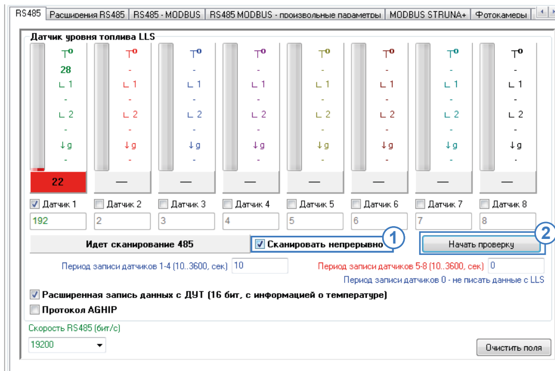
Рис.26. Проверка работы контроллера АвтоГРАФ с датчиками ТКАМ по протоколу LLS
