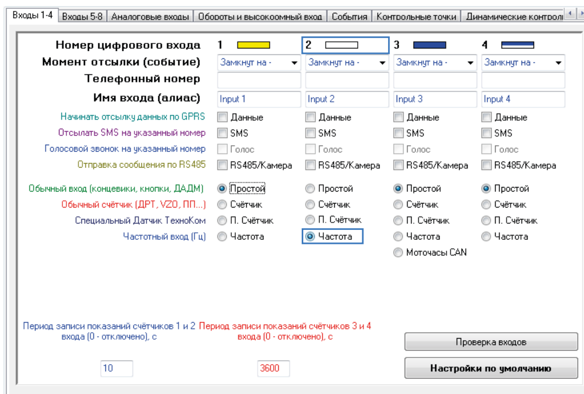
Рис.32. Настройка входа контроллера АвтоГРАФ в режим измерения частоты
