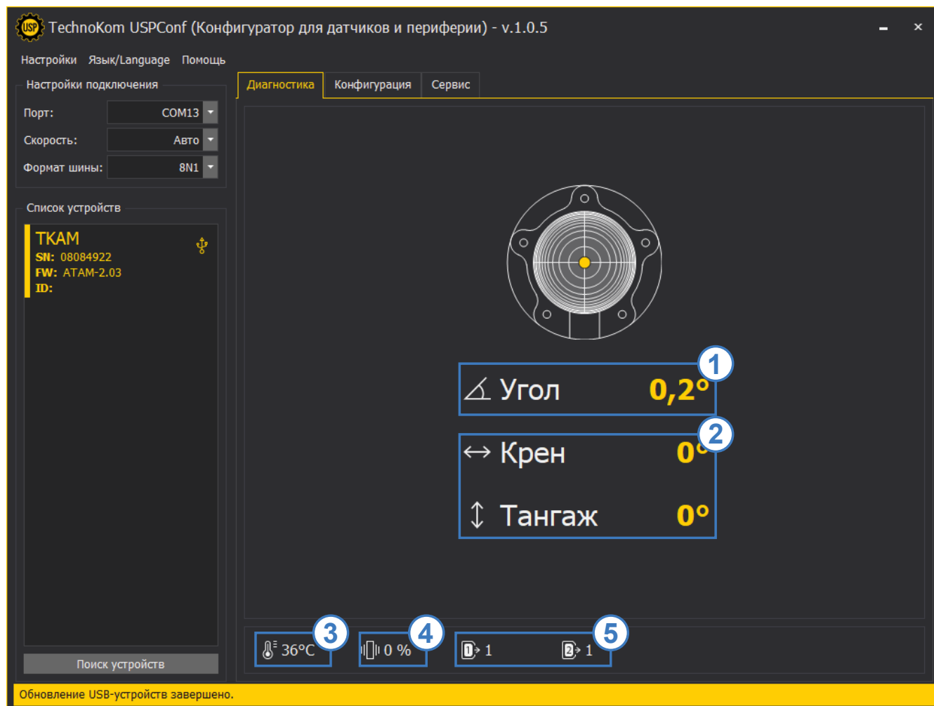
Рис.13. Диагностика датчика
