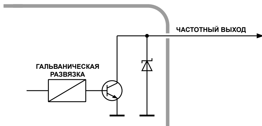
Рис.19. Внутренняя схема частотного выхода
