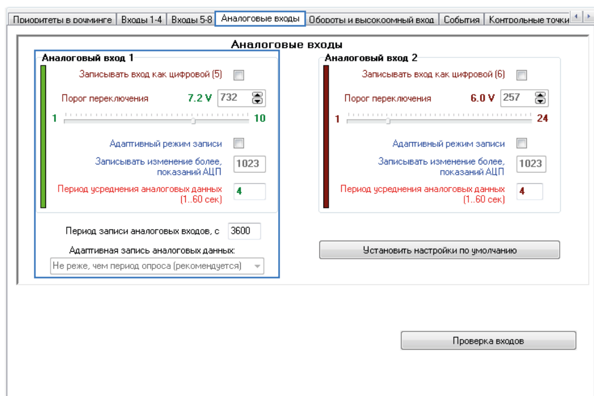
Рис.34. Пример настройки аналогового входа 1 контроллера АвтоГРАФ для подключения датчика ТКAM
