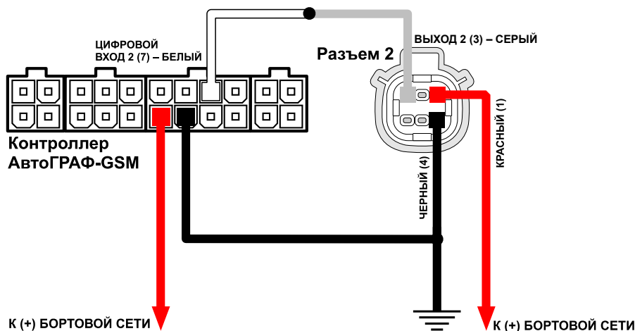
Рис.20. Структурная схема подключения частотного выхода
