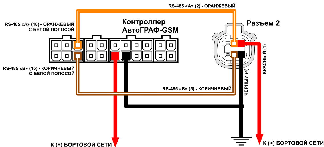
Рис.15. Схема подключения к шине RS-485
