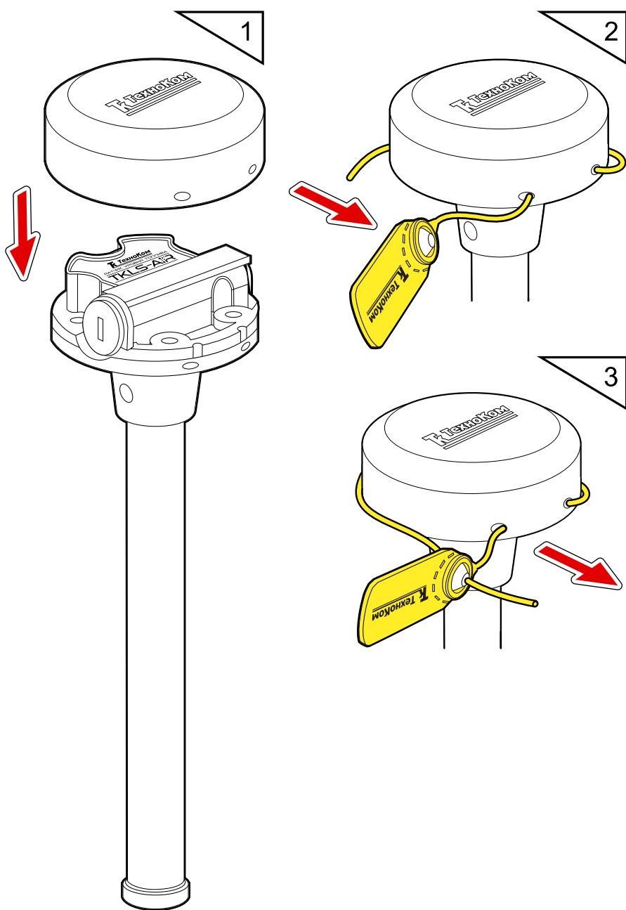
Рис.25. Пломбировка корпуса датчика.
