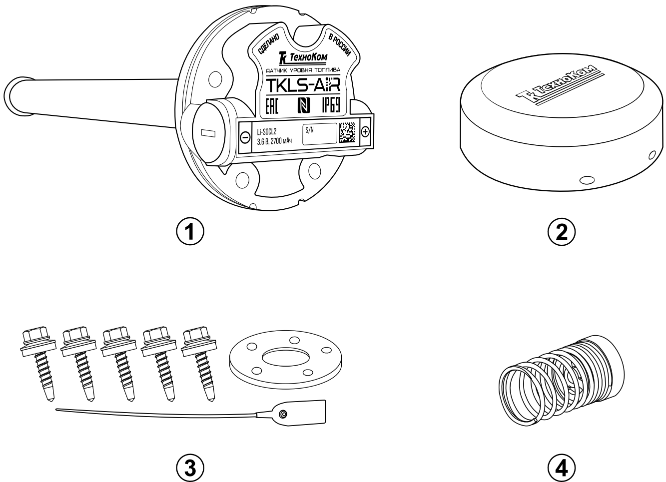
Рис.2. Комплект поставки.
