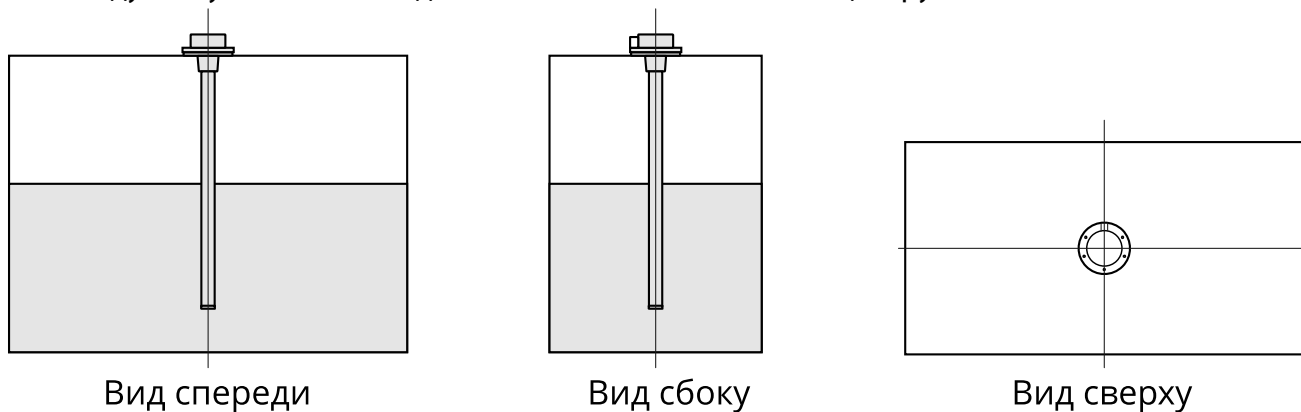
Рис.4. Рекомендованный вариант установки датчика в бак.
