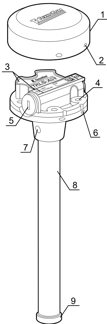
Рис.3. Составные части устройства.
