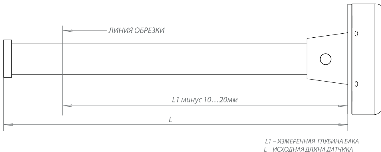
Рис.6. Обрезка измерительной части датчика.
