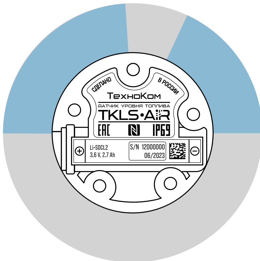
Рис.7. Рекомендованный вариант по расположению датчика.
