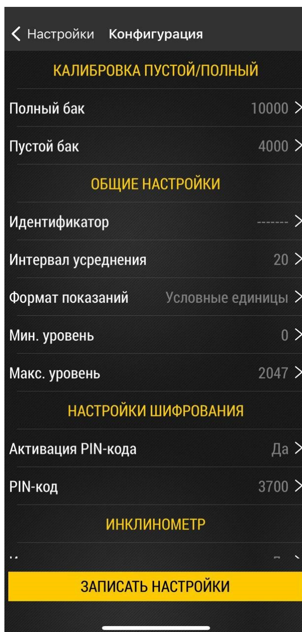
Рис.15. Настройки датчика.
